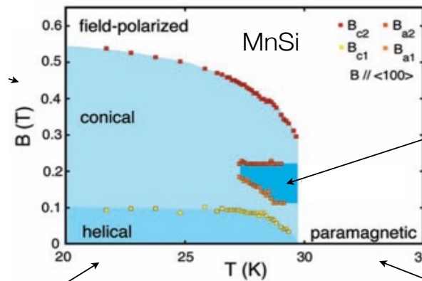
Skyrmion crystal
