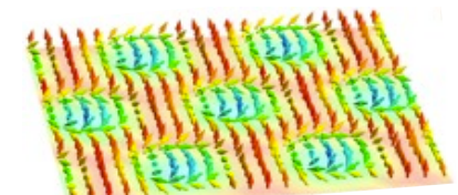
Skyrmion crystal
